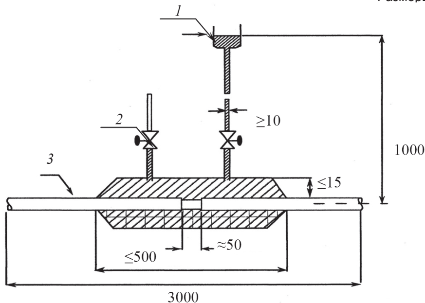
1 – резервуар с водой; 2 – вентиляционное отверстие; 3 – кабель
