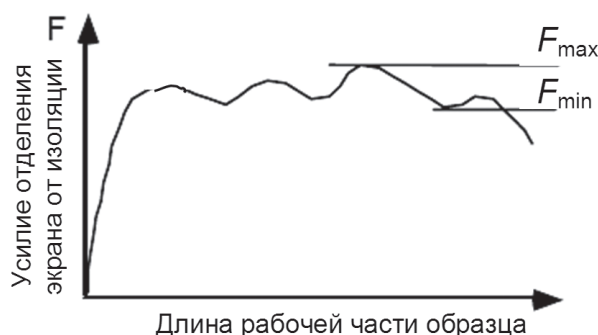
Рисунок 2 – Усилие отделения электропроводящего экрана от изоляции
