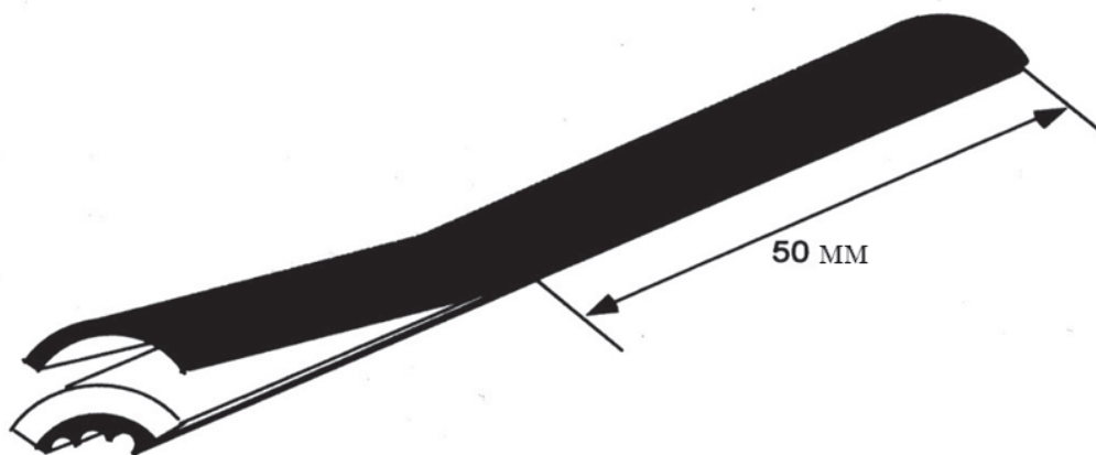
Рисунок 1 – Проверка отделяемости экструдированного электропроводящего экрана
