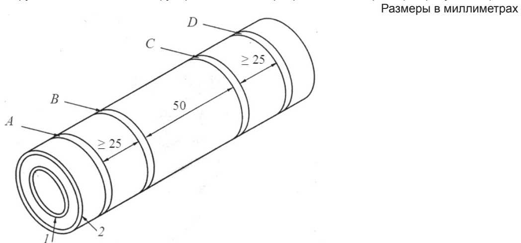
Рисунок Б.2 – Схема измерения электрического сопротивления экструдированного электропроводящего экрана по изоляции
